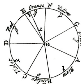
【図1】アイザック・ニュートン：『光学』命題 VI 問題 II、円周が7つの音階で分割される事を説明する図
